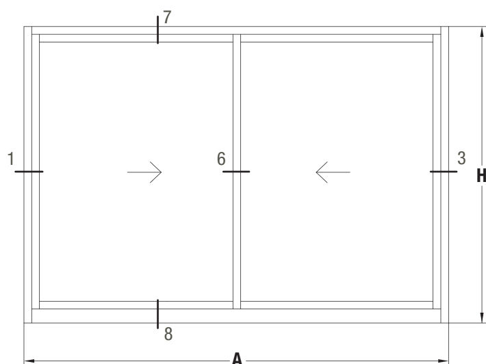
SECCIÓN 1-6-3
