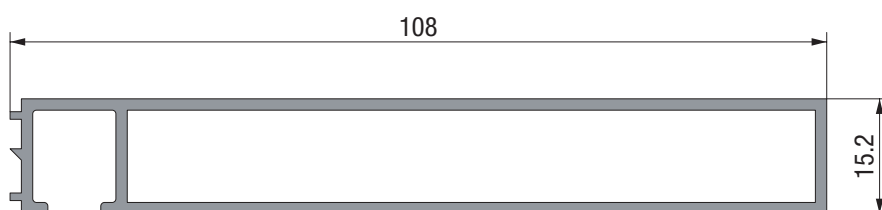
6079 0,994 Kg/m
