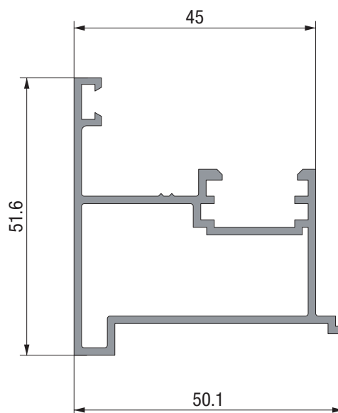
6224 0,794 Kg/m
