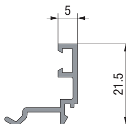
6220 0,176 Kg/m
