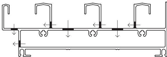
ESQUEMA DESAGÜES UMBRAL 3 GUIAS
