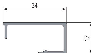
8707 0,264 Kg/m
