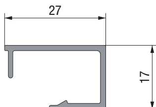
8706 0,240 Kg/m
