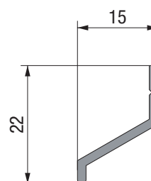
5746 0,127 Kg/m
