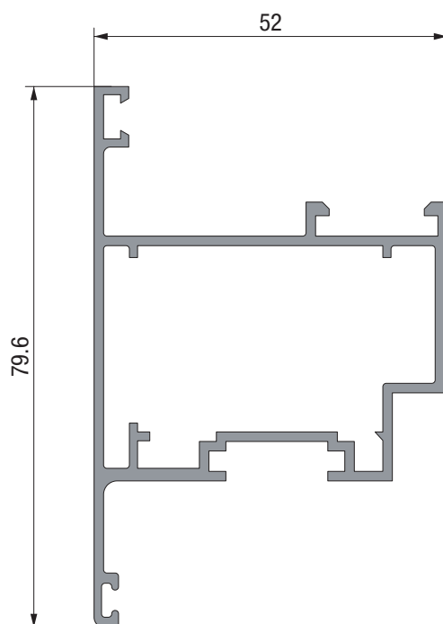
6258 1,061 Kg/m
