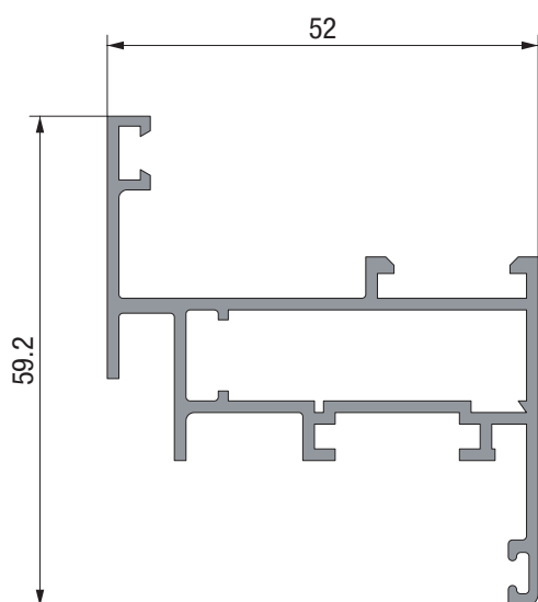
6215 0,864 Kg/m
