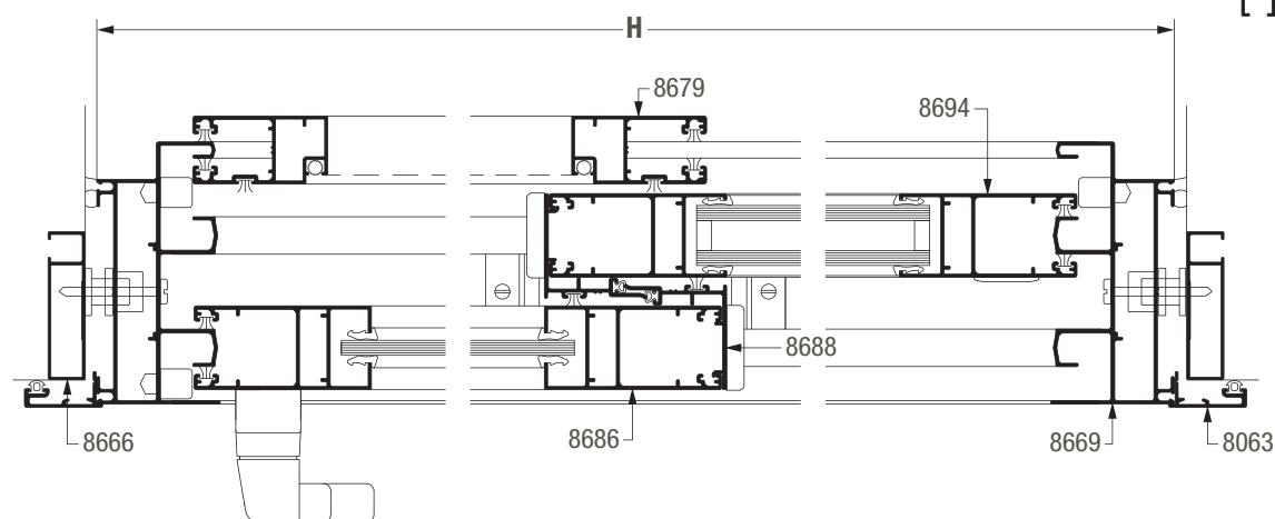
SECCION 1-2-3
