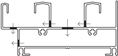
ESQUEMA DESAGÜES UMBRAL 2 GUIAS
