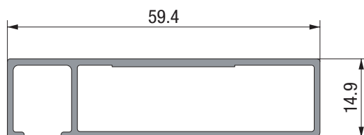
8666 0,478 Kg/m
